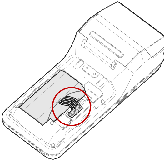
Figure 6 배터리 삽입하기 - 2
