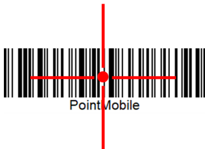
Figure 32 바코드 스캔하기
