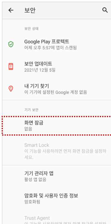
Figure 26 화면 잠금
