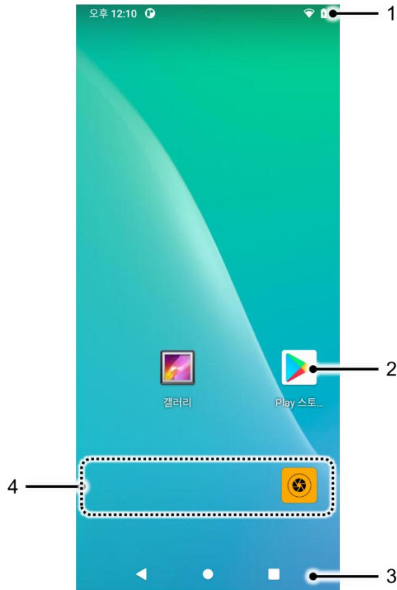
Figure 17 홈 화면
